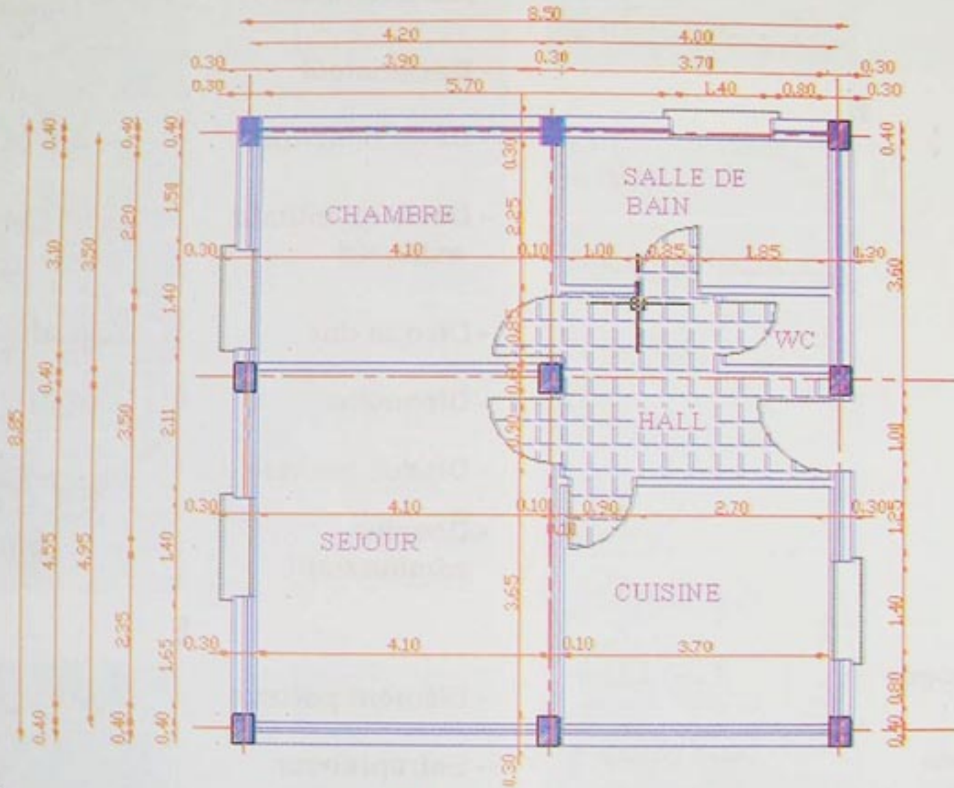
Plan de répartition d'une cellule F2
