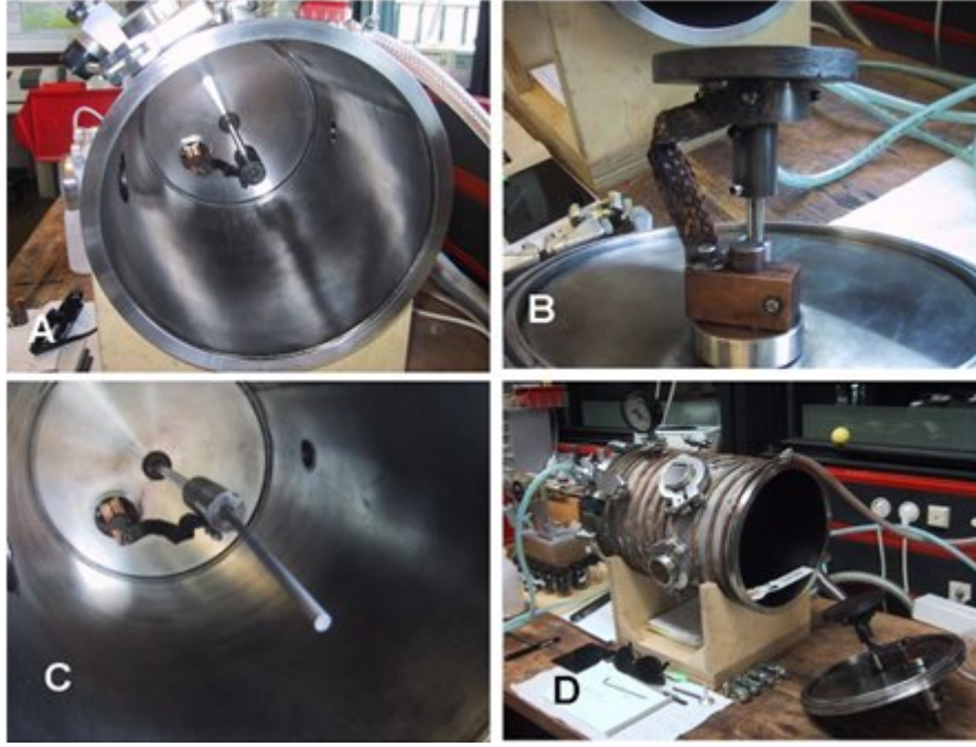
شكل (14): صور تبين مفاعل إنتاج الأنابيب النانوية (Nanotubes Reactor) .
