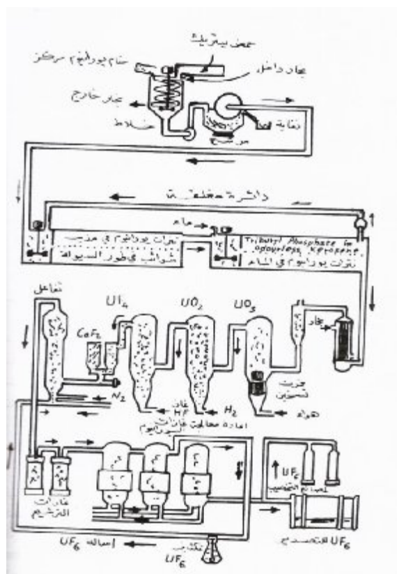
الشكل - 2 المناجم وعمليات تحضير UF_6 من U_3O_8 (الكعكة الصفراء)
