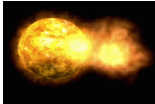
الرياح الشمسية
