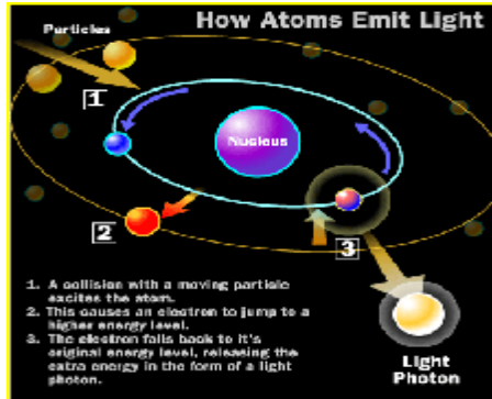
انبعاث الفوتونات
