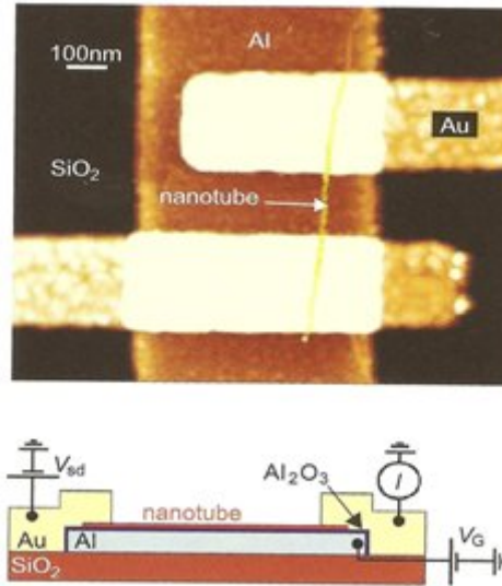
شكل (9) : أحد التطبيقات الالكترونية بحيث أن صورة المجهر الالكتروني (STM) توضح ترانزستور من نوع-CN FET
