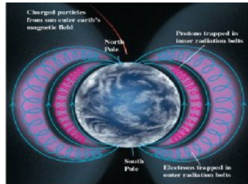
أحزمة فان ألن الإشعاعية
