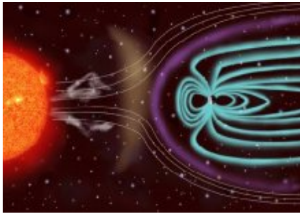
تأثير المجال المغناطيسي الأرضي بالرياح الشمسية
