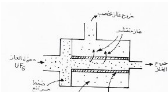
الشكل 6- تخصيب اليورانيوم باستخدام تقنية الانتشار الغازي
