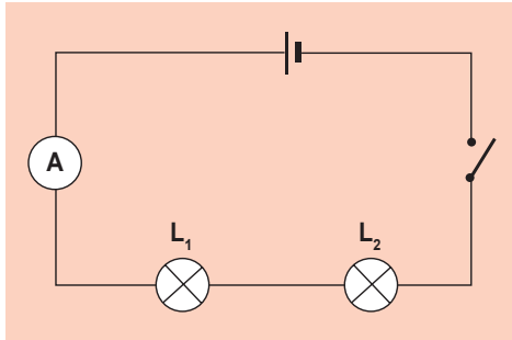
■ وثيقة 4 – مخطط الدارة
