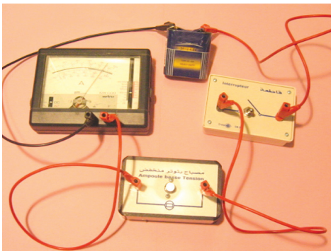
■ وثيقة 6 - تركيب الدارة
