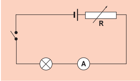
■ وثيقة 3 - مخطط الدارة
