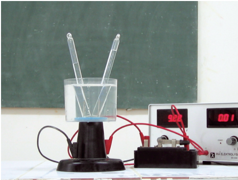
■ وثيقة 2 – تجربة التحليل الكهربائي
