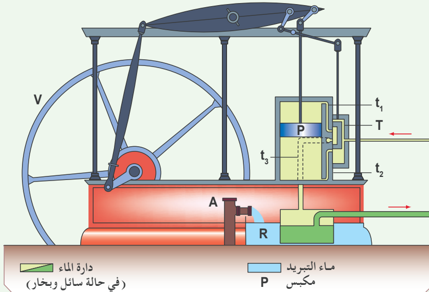
رسم تخطيطي لماكينة واط Watt
