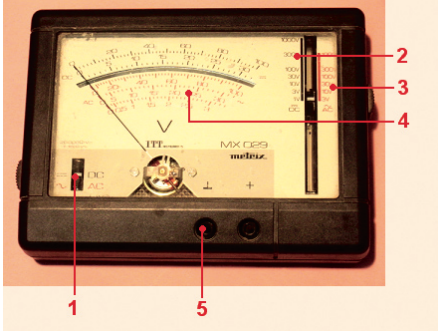
■ وثيقة 1 - فولط متر
