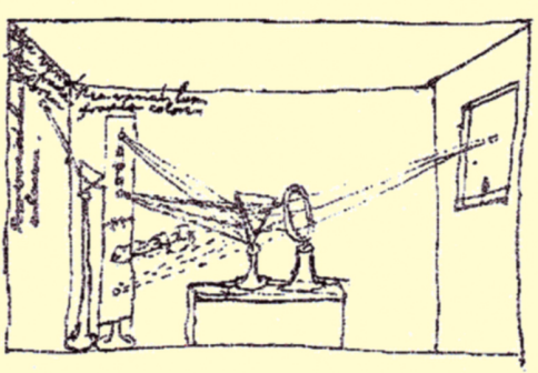
■ وثيقة 7 - رسم تخطيطي قدمه نيوتن لتجربته المشهورة
