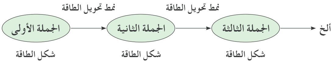
■ وثيقة 2 - نموذج السلسلة الطاقوية
