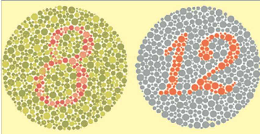
■ وثيقة 2 - صورتان لاختبار عمى الألوان
