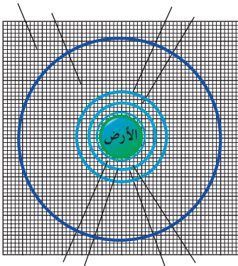
■ وثيقة 5 - بيان تخطيطي لطبقات الغلاف الجوي
