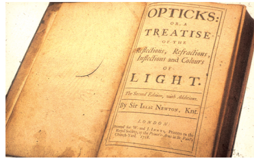
■ وثيقة 6 - كتاب إسحاق نيوتن الذي يبين فيه العلاقة بين الضوء واللون
