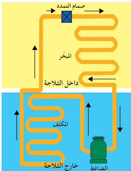
■ وثيقة 3 - مخطط لقسامي الثلاجة
