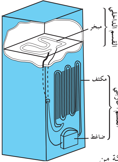
■ وثيقة 2 - قسما الثلاجة
