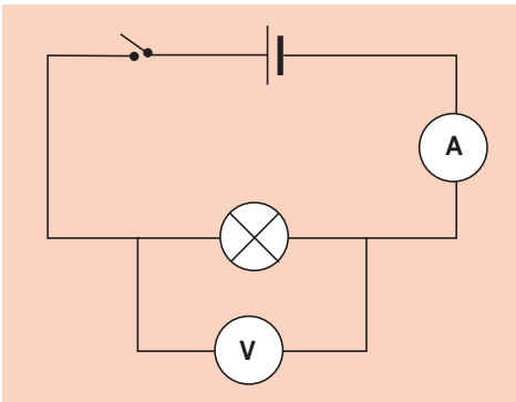
■ وثيقة 5 - المخطط الكهربائي
