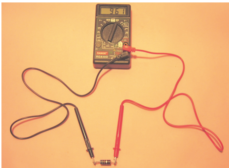
■ وثيقة 3 - القياس المباشر لقيمة المقاومة
