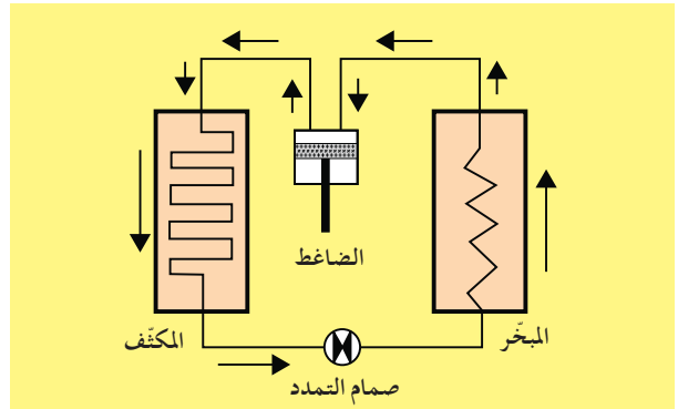
■ وثيقة 4 - مخطط لدورة الغاز
