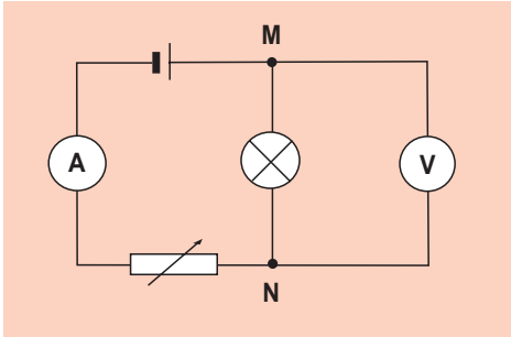
■ وثيقة 7 - مخطط الدارة
