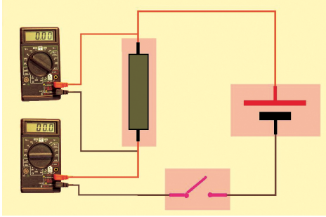
■ وثيقة 2 - توصيلان مختلفان لمتعدد قياسات
