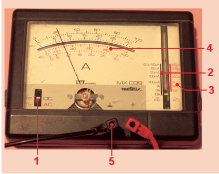
■ وثيقة 1 - أمبير متر
