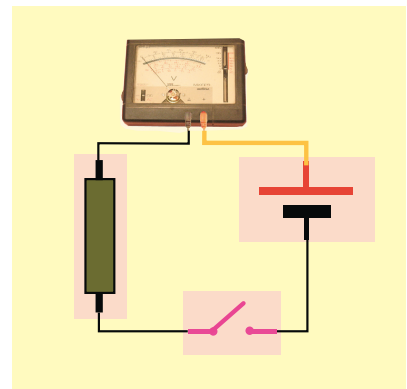
■ وثيقة 2 - توصيل أمبير متر في دارة كهربائية
