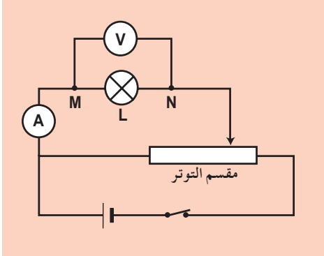
■ وثيقة 6 - مخطط الدارة
