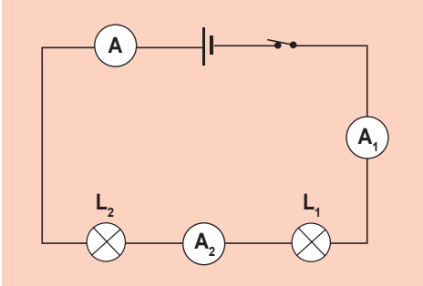
■ وثيقة 3 - المخطط الكهربائي
