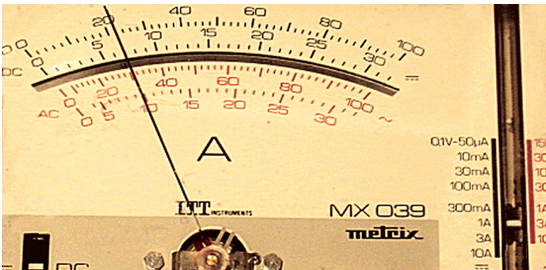
■ وثيقة 3 - ميناء الأمبير متر
