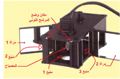
■ وثيقة 1 - منبع ضوئي
