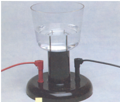
■ وثيقة 4 - وعاء التحليل الكهربائي
