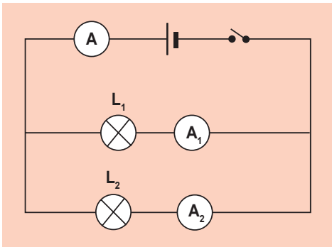
■ وثيقة 4 - المخطط الكهربائي
