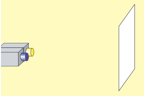
■ وثيقة 1 - تركيب ضوئين
