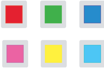
■ وثيقة 3 - مرشحات لونية
