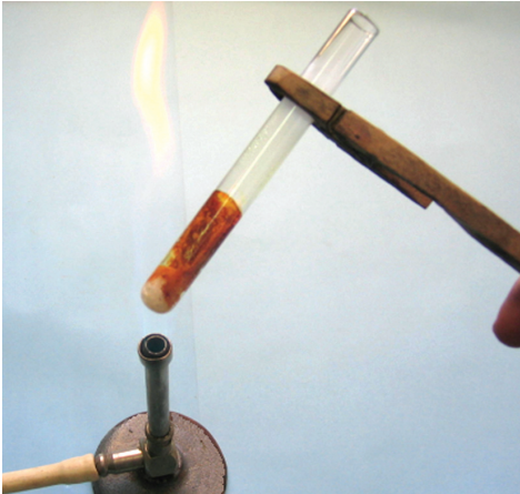
■ وثيقة 2 - تسخين السكر
