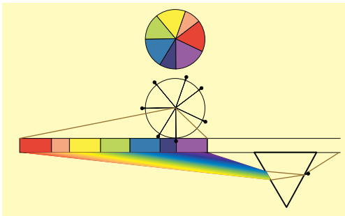
■ وثيقة 9 - المجموعات اللونية السبعة للضوء الأبيض عند نيوتن
