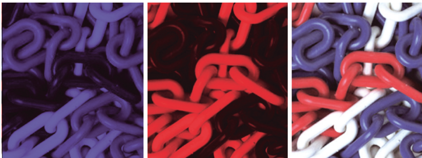
■ وثيقة 2 - لون الجسم في حالات مختلفة
