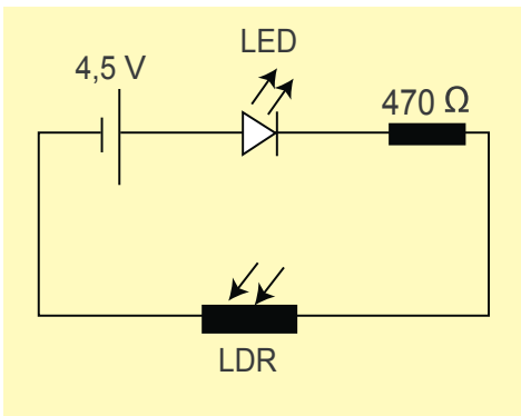
■ وثيقة 10 – المخطط الكهربائي
