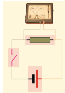
■ وثيقة 2 - توصيل فولط متر في دارة كهربائية
