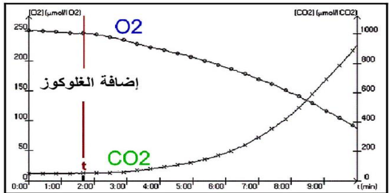
الوثيقة 1 : تطور تركيز الغازات التنفسية في وجود خلايا الخميرة
